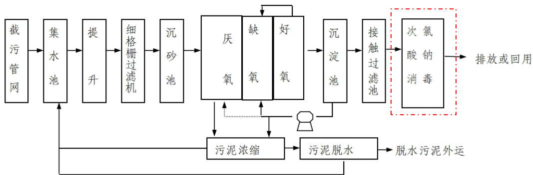
图 4.1-2 一期工程变动后生产工艺流程及产污环节图
